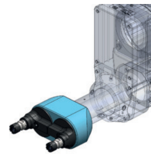
Têtes multibroches Mehrs spindleköpfe
